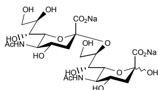
N -Acetylneuraminic acid, dimer (α, 2→8), disodium salt
