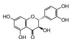
(+)- trans -Taxifolin
