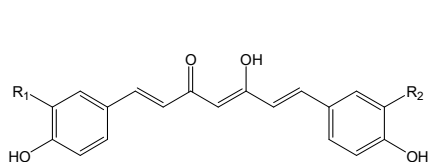
Curcumin 1 R_1=R_2=OCH_3 Curcumin 2 R_1=H, R_2=OCH_3 Curcumin 3 R_1=R_2=H
